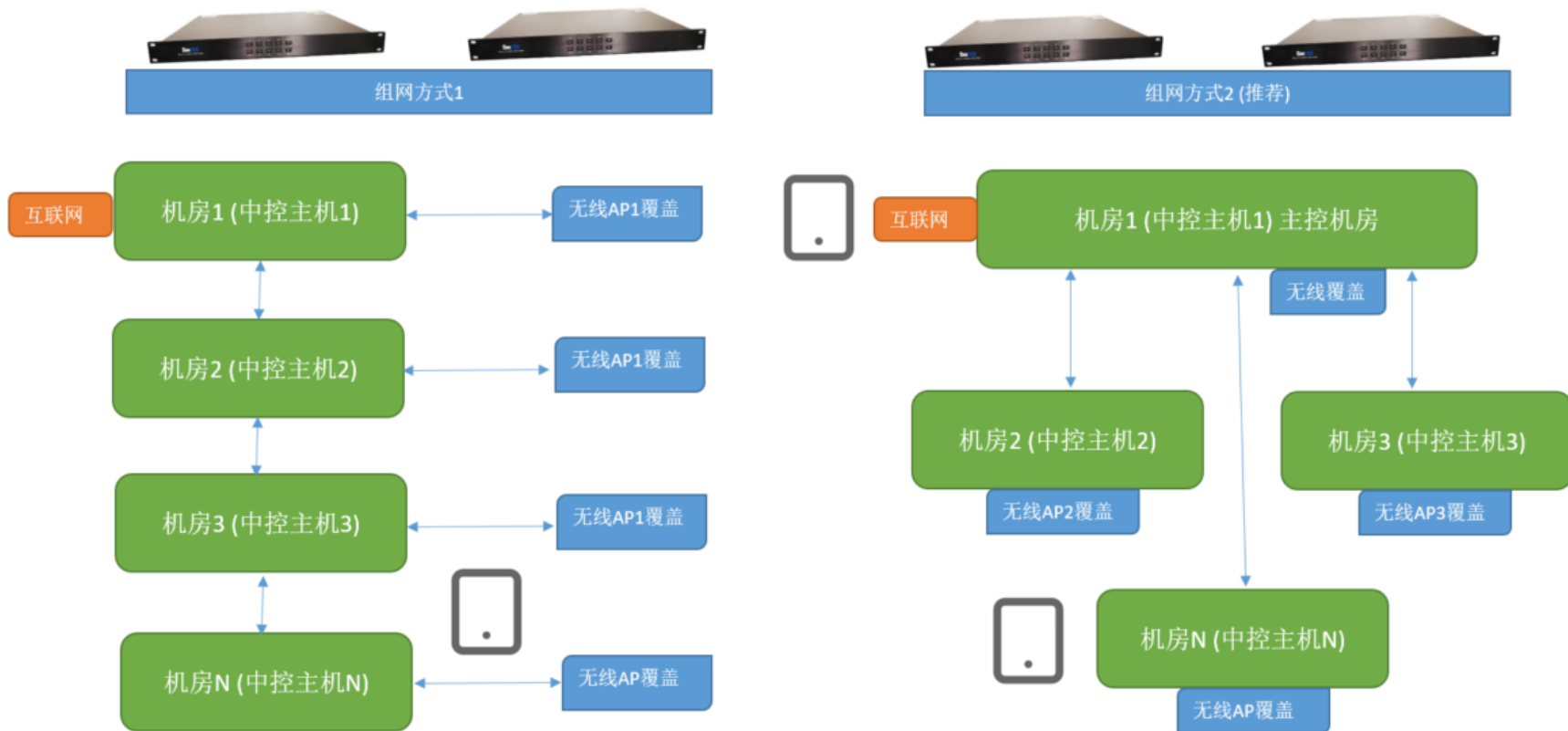
SimFAS中控系统 -多层展厅(多中控)集控 布线原理图
